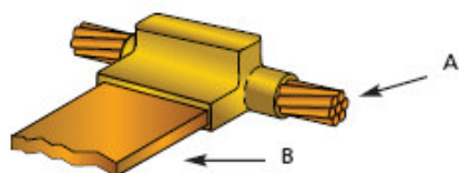
LE – Horizontálne pripojenie kábla na ploché výstupky
